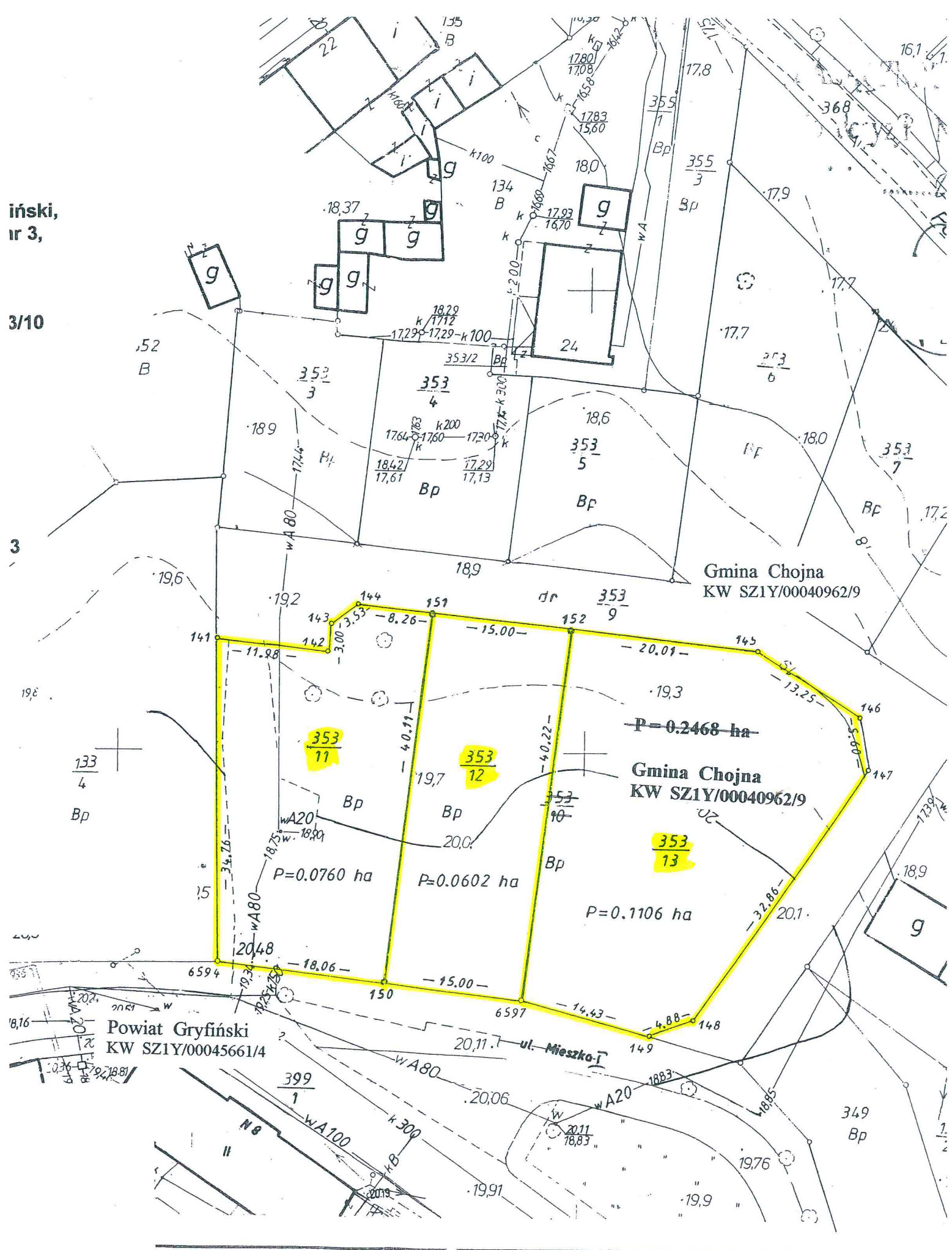
Mapa zasadnicza 1:500
